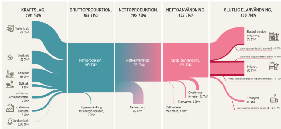
Figur 1 Sankey diagram av prognosticerade elflöden inom Sveriges elsystem 2027, TWh. Anm. Dessutom kan bruttoanvändning sägas vara en kombination av nettoanvändning och egenanvändning för energiproduktion.
